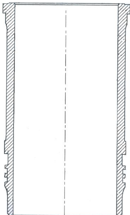
Рис. 1. Гильза 236-1002021-А5 старого исполнения
