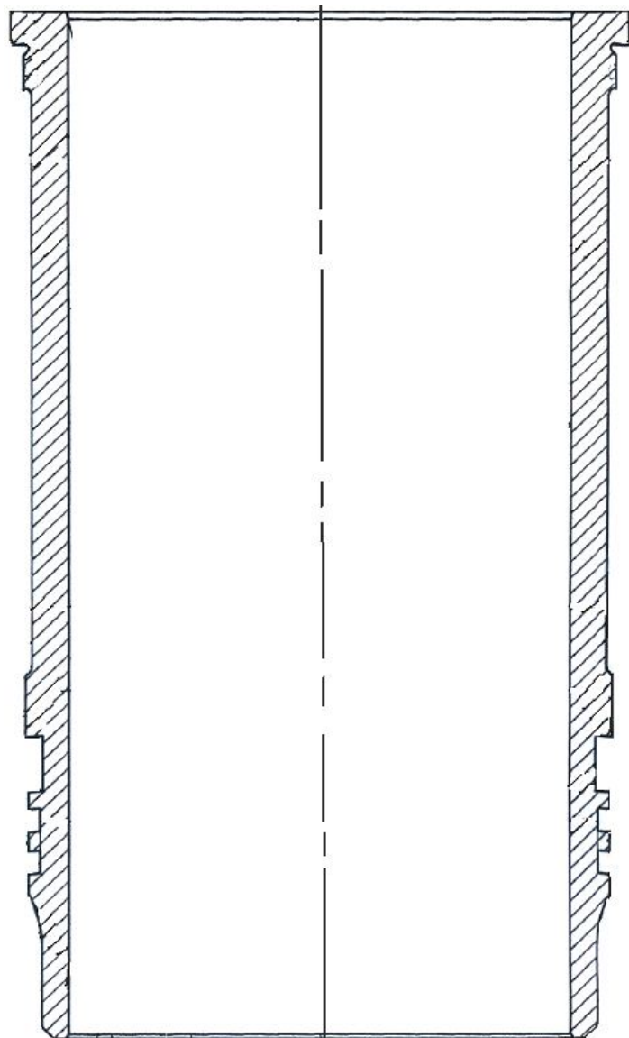
Рис. 7. Гильза 7511.1002021-01 старого исполнения
