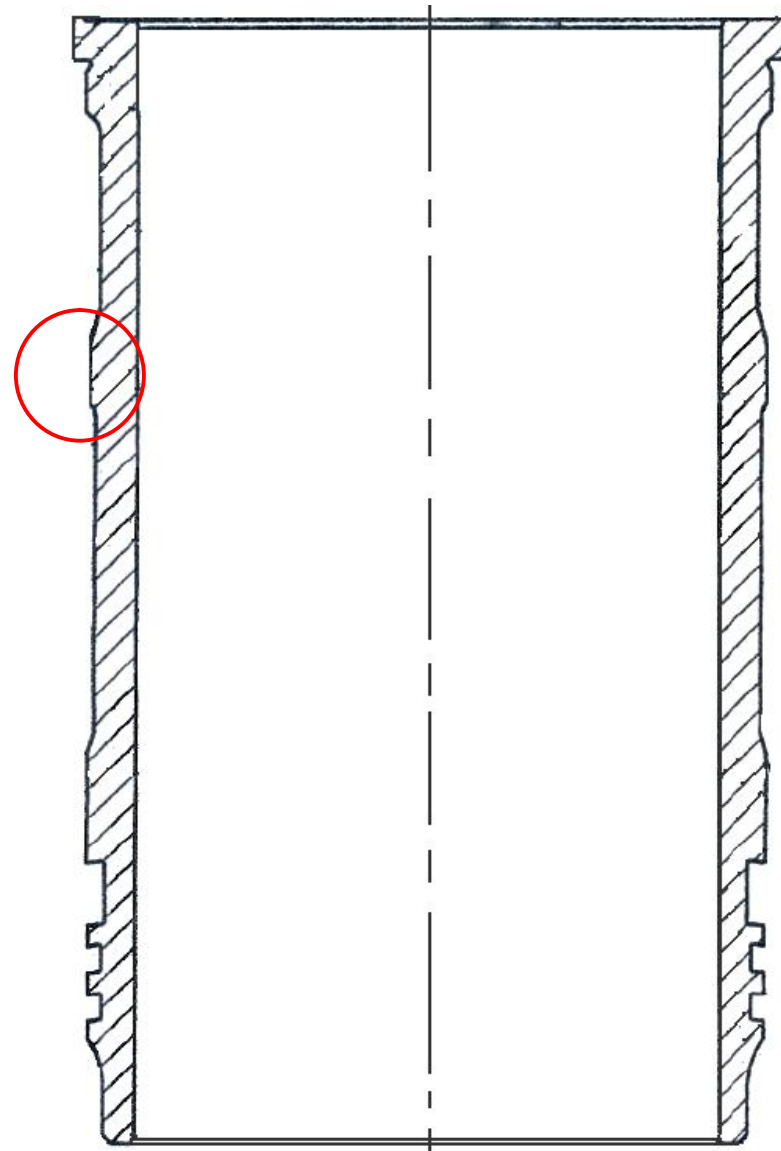
Рис. 8. 7511.1002021-01 нового исполнения
