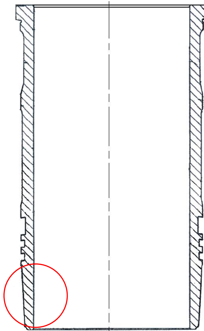
Рис. 4. Гильза 236-1002021-Б2 нового исполнения
