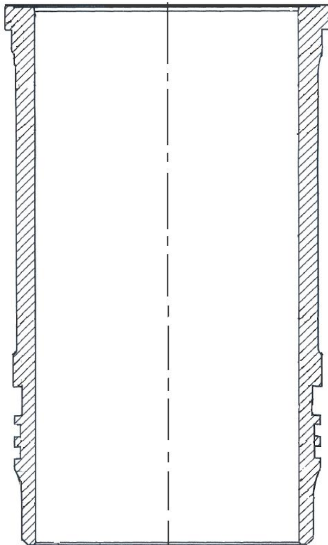
Рис. 9. Гильза 240-1002021-Б4 старого исполнения
