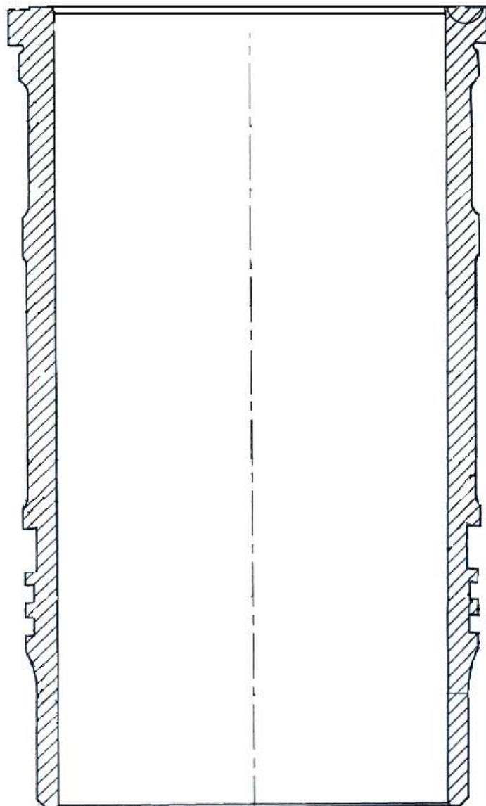
Рис. 3. Гильза 236-1002021-Б2 старого исполнения
