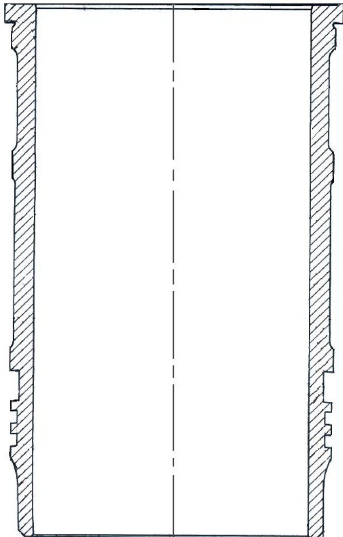
Рис. 5. Гильза 7511.1002021-10 старого исполнения
