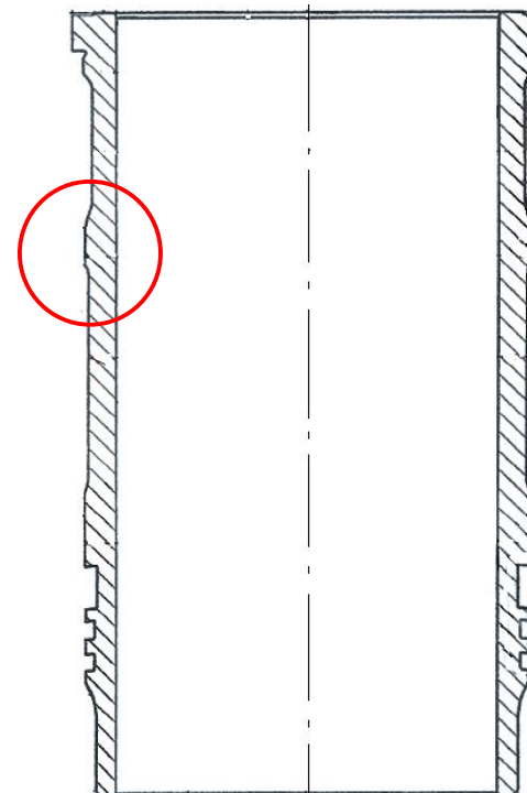
Рис. 2. Гильза 236-1002021-А5 нового исполнения
