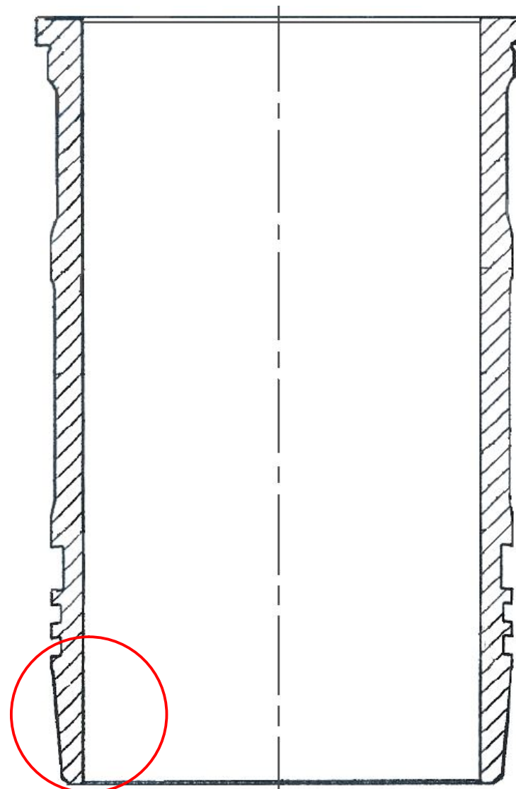
Рис. 6. 7511.1002021-10 нового исполнения
