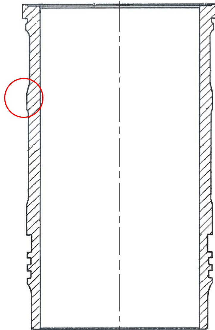
Рис. 10. Гильза 240-1002021-Б4 нового исполнения
